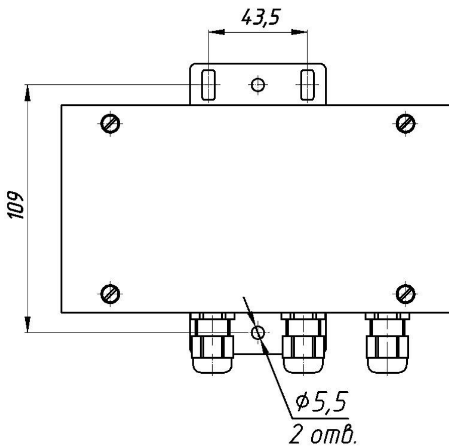
б) на стене
