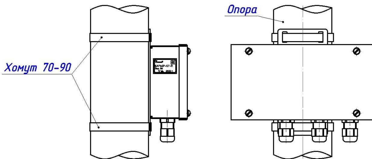
а) на опоре
